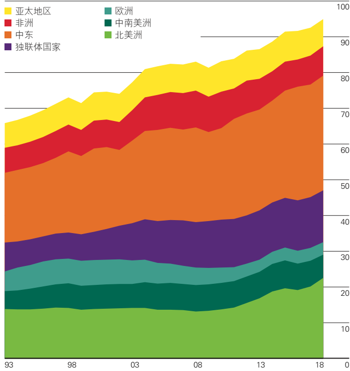
石油: 分区域产量 (单位: 百万桶/日)
