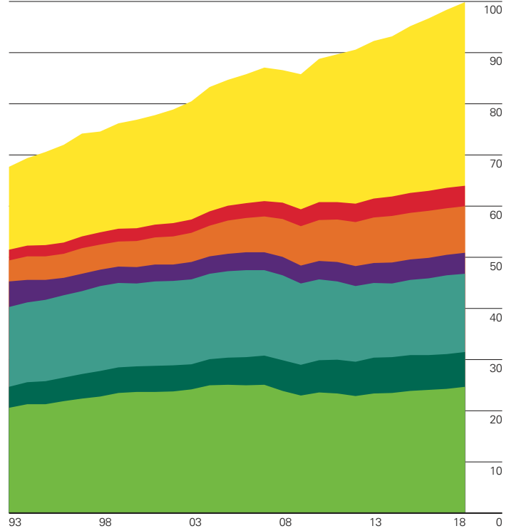
石油: 分区域消费量 (单位: 百万桶/日)
