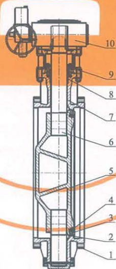
图7 对夹式衬胶(氟)中心蝶阀
