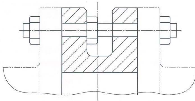
图 5 U形截面对夹式
