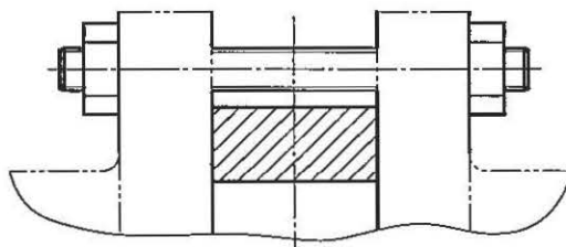
图 3 无法兰对夹式
