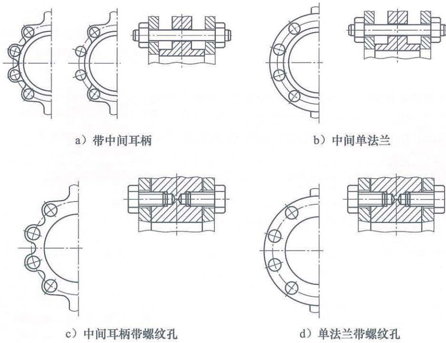
图 4 单法兰或耳柄对夹式
