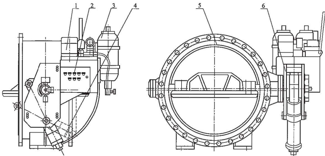
图9 凸耳对夹式连接蝶阀
